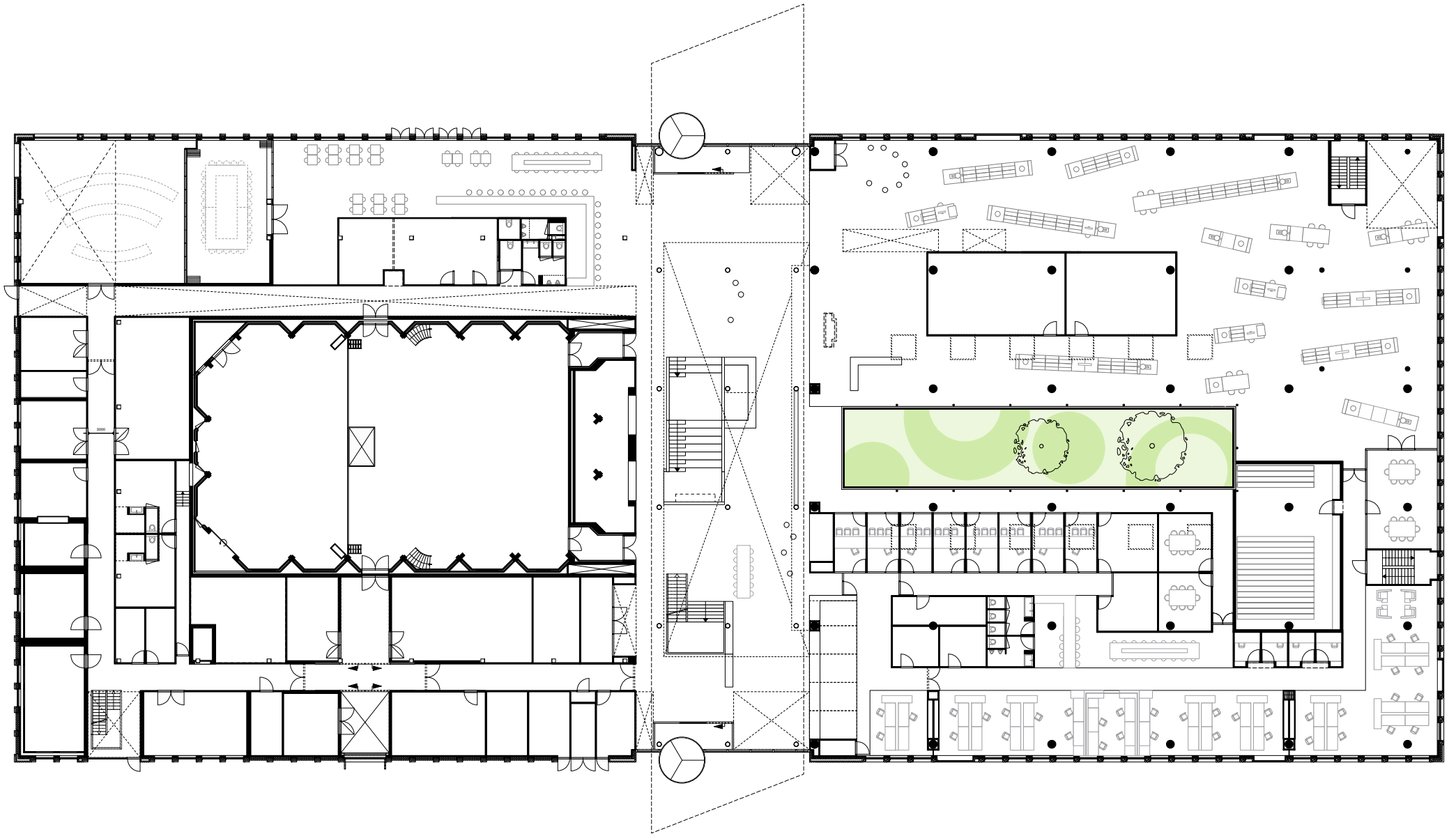
Plattegrond fase 1 en fase 2 gereed
