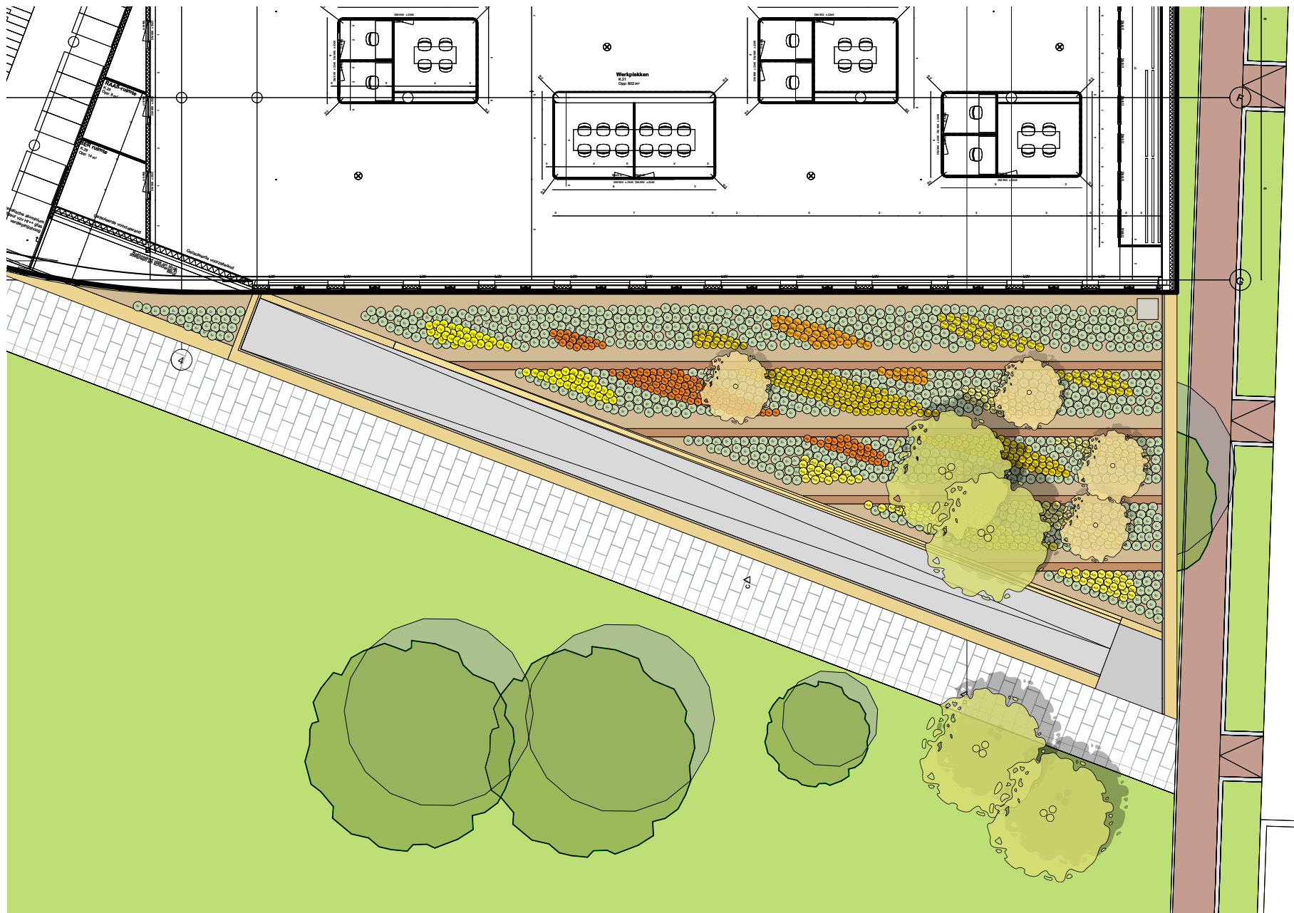
Kielzog Hoogezand Plattegrond hellingtuin
