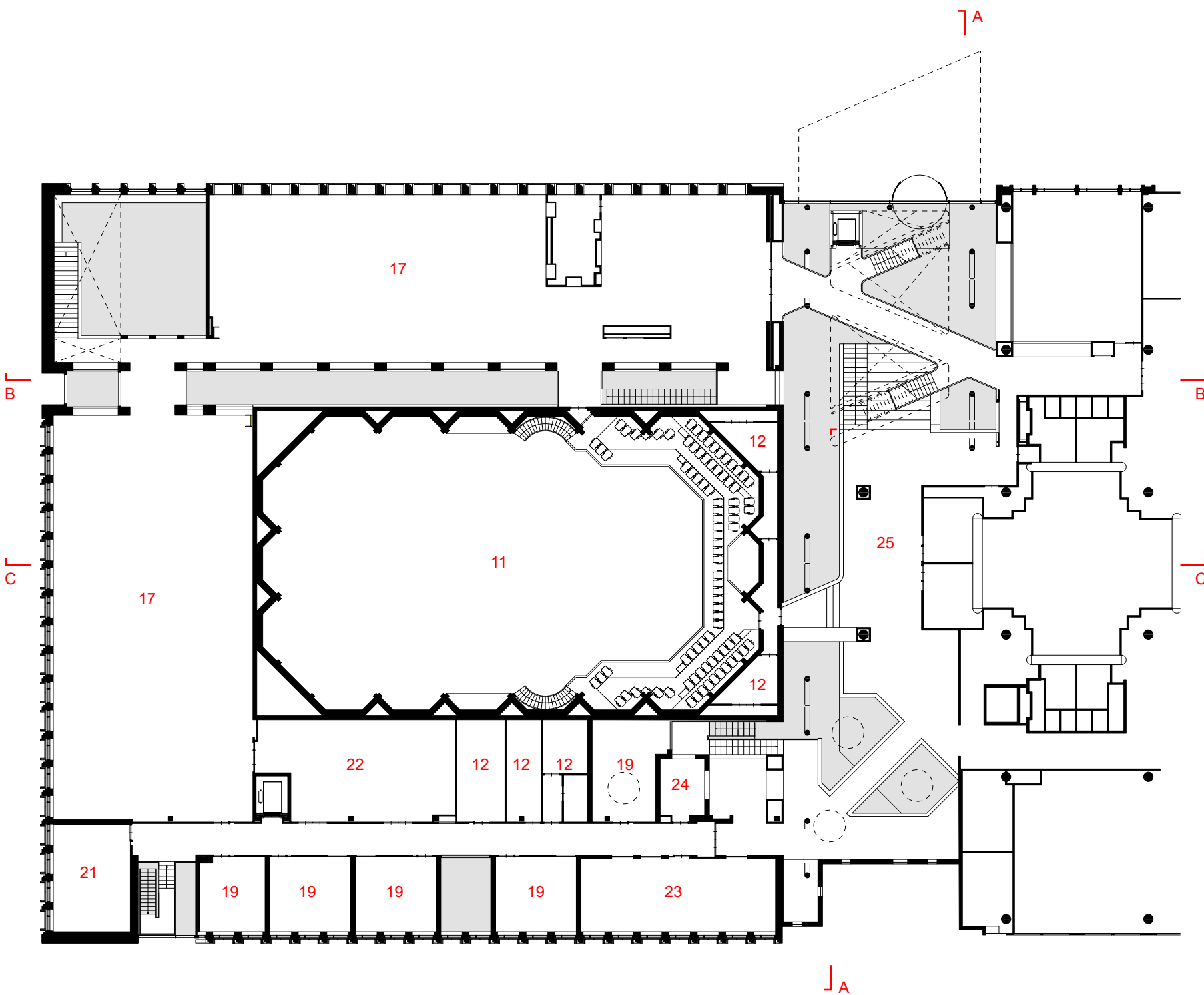
Plattegrond eerste verdieping
