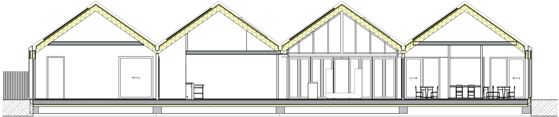
Doorsnede AA
