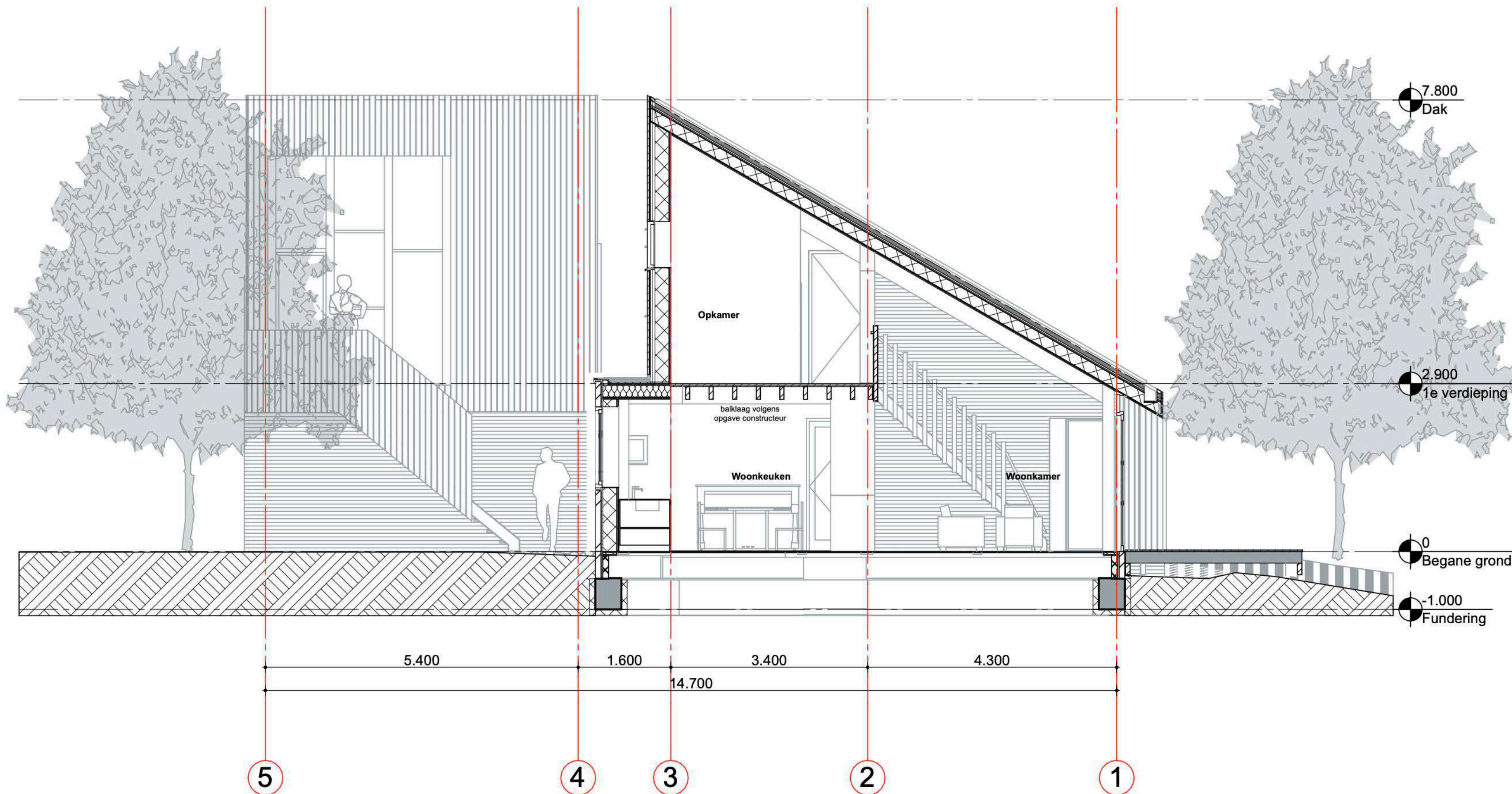
Doorsnede A-A Woonhuis
