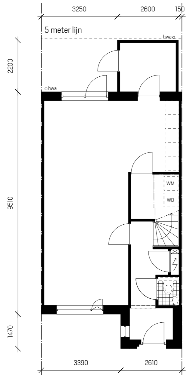
Begane grond
